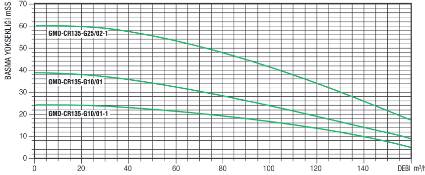
PERFORMANS EĞRİLERİ
