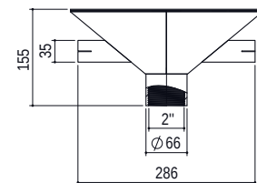
Yandan görünüş
